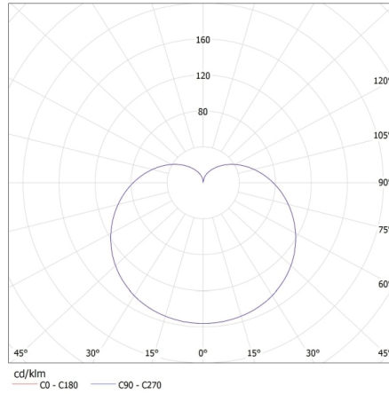
KANLUX S.A. (kat 23042) BILO 5W T SMD E14-WW / Krzywa rozsyłu światła (biegunowo)
