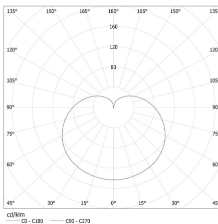
KANLUX S.A. (kat 27270) IQ-LED A60 5,5W-WW / LDC (Polar)
