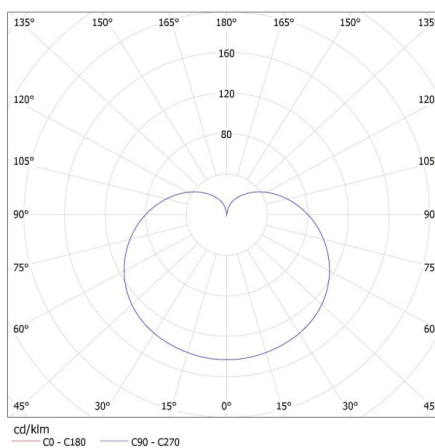
KANLUX S.A. (kat 27271) IQ-LED A60 5,5W-NW / LDC (Polar)
